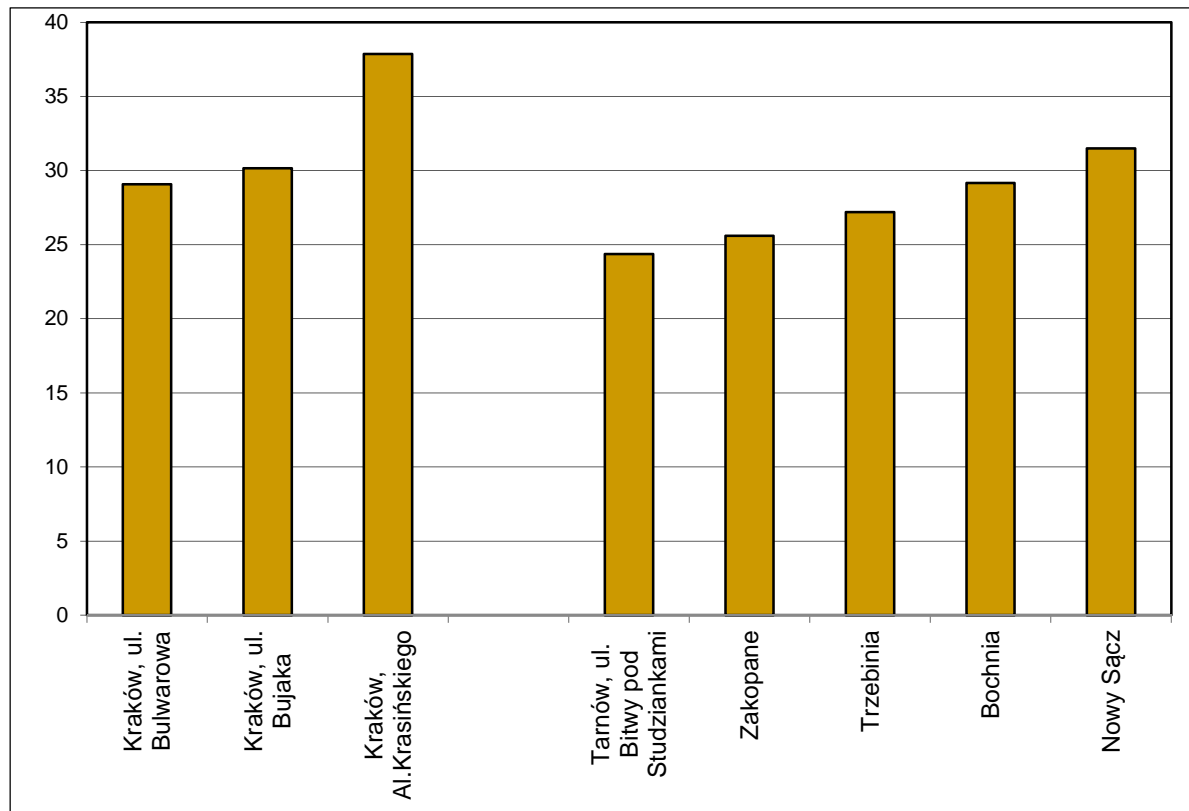
Wykres 7. Roczne stężenia pyłu zawieszonego PM 2,5 (µg/m 3 ) na stanowiskach wykorzystanych do oceny
