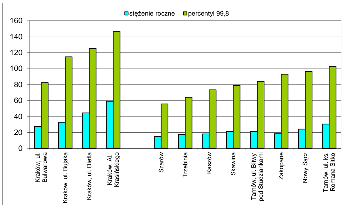
Wykres 2. Stężenia dwutlenku azotu ( \mu\text{g}/\text{m}^3 ) wykorzystane do oceny – pomiar automatyczny
