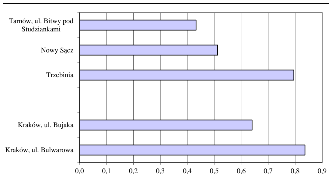
Wykres 9. Roczne stężenia kadmu (ng/m 3 ) na stanowiskach wykorzystanych do oceny – pomiar manualny
