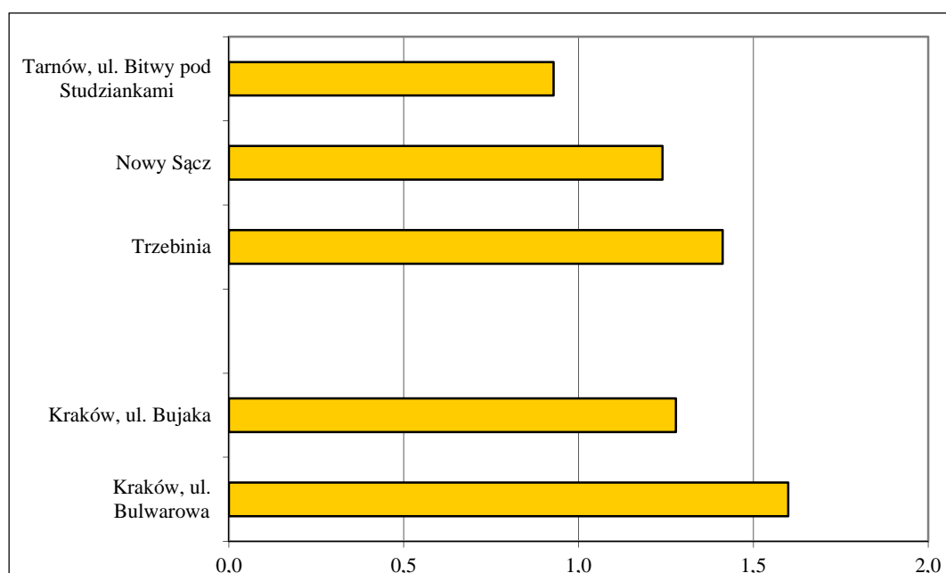
Wykres 10. Roczne stężenia niklu (ng/m 3 ) na stanowiskach wykorzystanych do oceny – pomiar manualny
