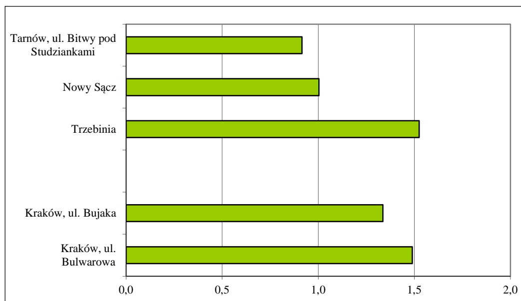
Wykres 8. Roczne stężenia arsenu (ng/m 3 ) na stanowiskach wykorzystanych do oceny – pomiar manualny
