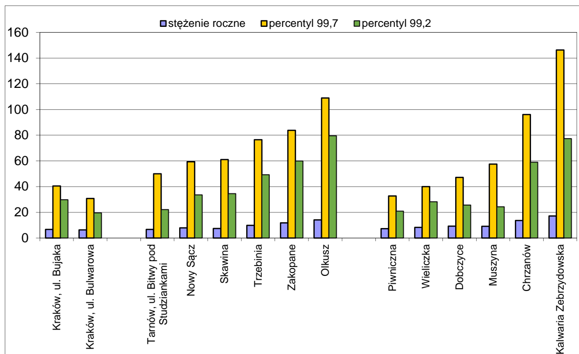
Wykres 1. Stężenia dwutlenku siarki ( \mu\text{g}/\text{m}^3 ) wykorzystane do oceny – pomiar automatyczny
