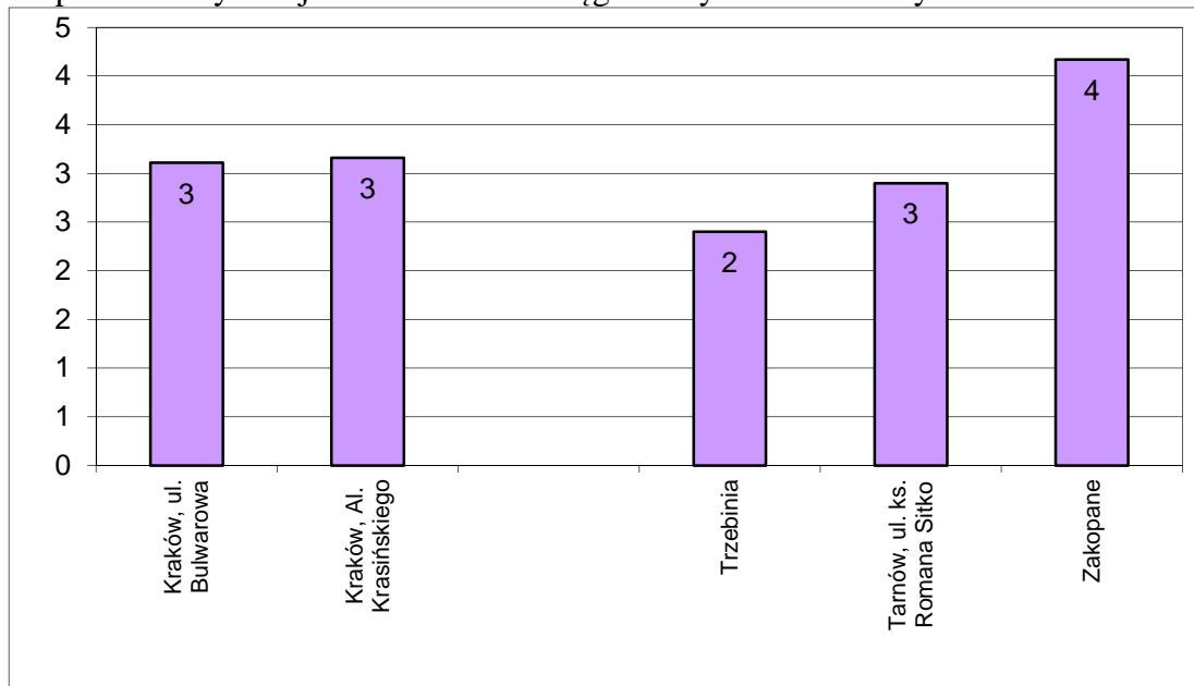
Wykres 3. Maksymalne stężenia tlenku węgla średnie 8 godzinne spośród średnich kroczących ( \text{mg}/\text{m}^3 ) wykorzystane do oceny – pomiar automatyczny
