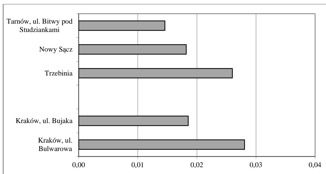
Wykres 6. Roczne stężenia ołowiu ( \mu\text{g}/\text{m}^3 ) na stanowiskach wykorzystanych do oceny – pomiar manualny
