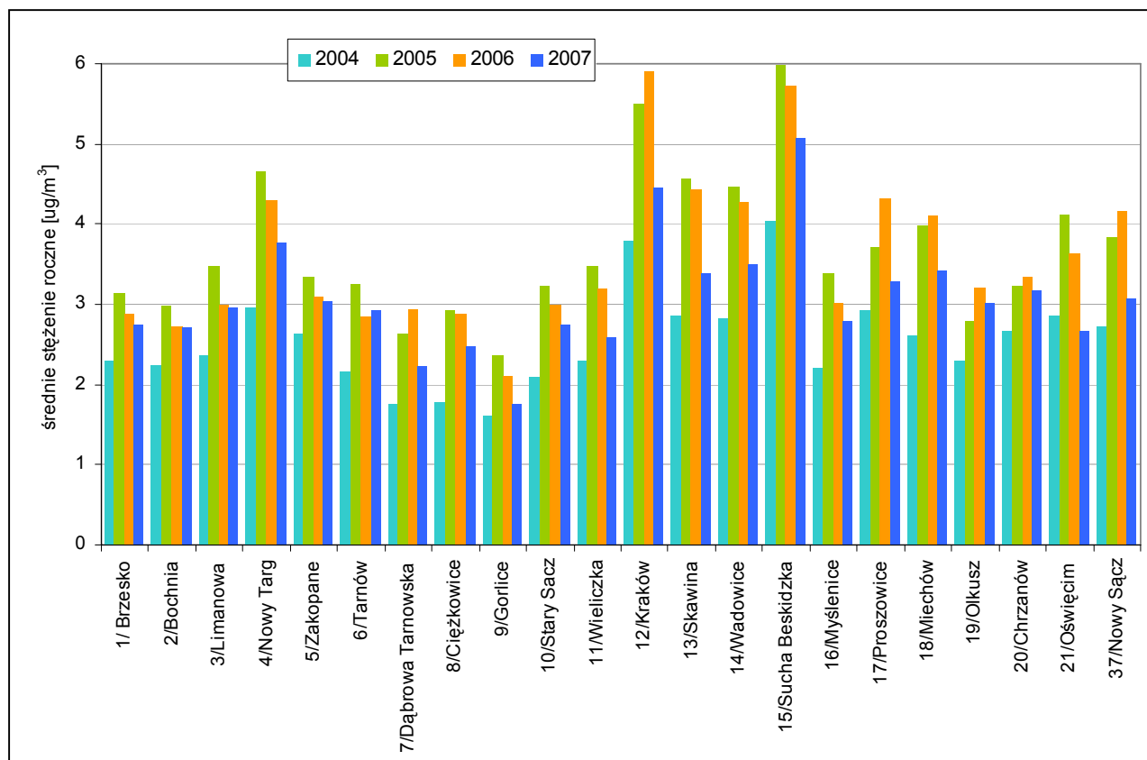
Rys.5. Porównanie stężeń średniorocznych benzenu na poszczególnych stanowiskach w latach 2004-2007 w województwie małopolskim.
