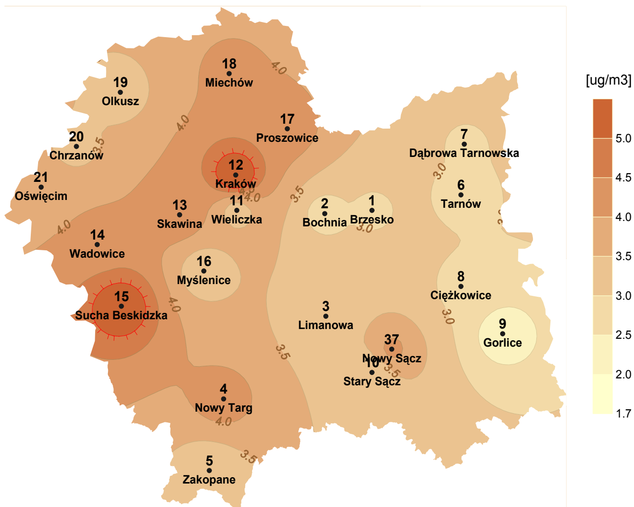
Rys.2. Rozkład średnich stężeń benzenu na obszarze województwa małopolskiego w 2007 roku.
