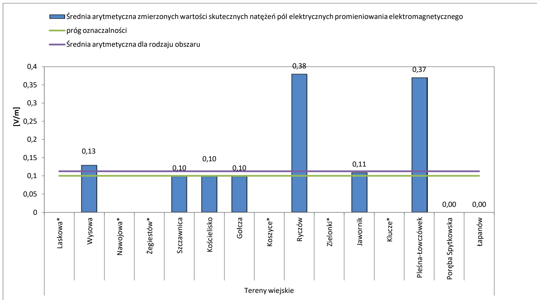
Wykres 3. Wyniki pomiarów pól elektromagnetycznych w 2018 roku w województwie małopolskim dla kategorii tereny wiejskie
