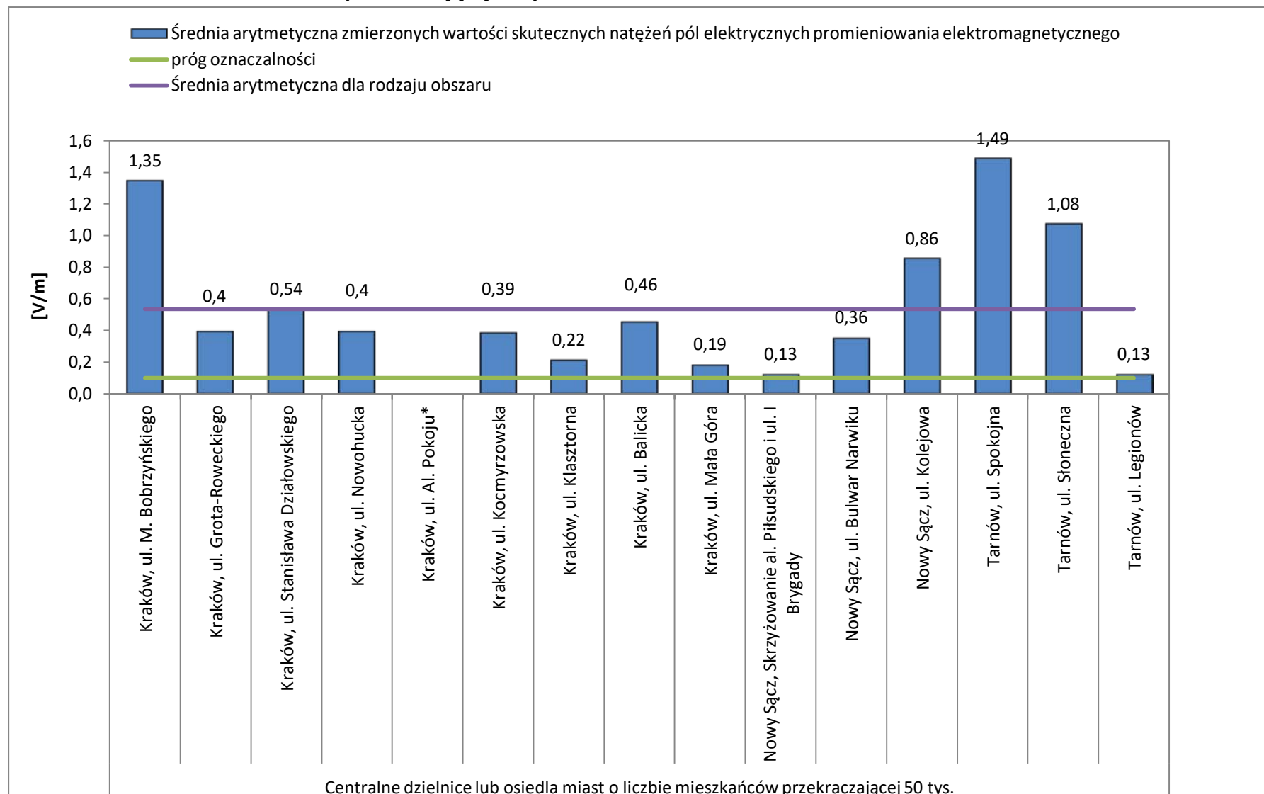
Wykres 1. Wyniki pomiarów pól elektromagnetycznych w 2018 roku w województwie małopolskim dla kategorii centralne dzielnice lub osiedla miast o liczbie mieszkańców przekraczającej 50 tys.
